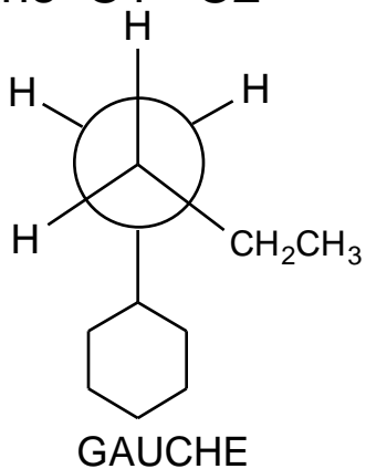
1-Cyclohexylbutane C1 - C2
