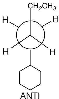
1-Cyclohexylbutane C1 - C2
